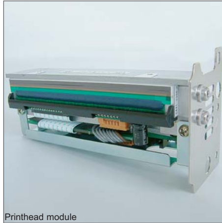
Printhead module
